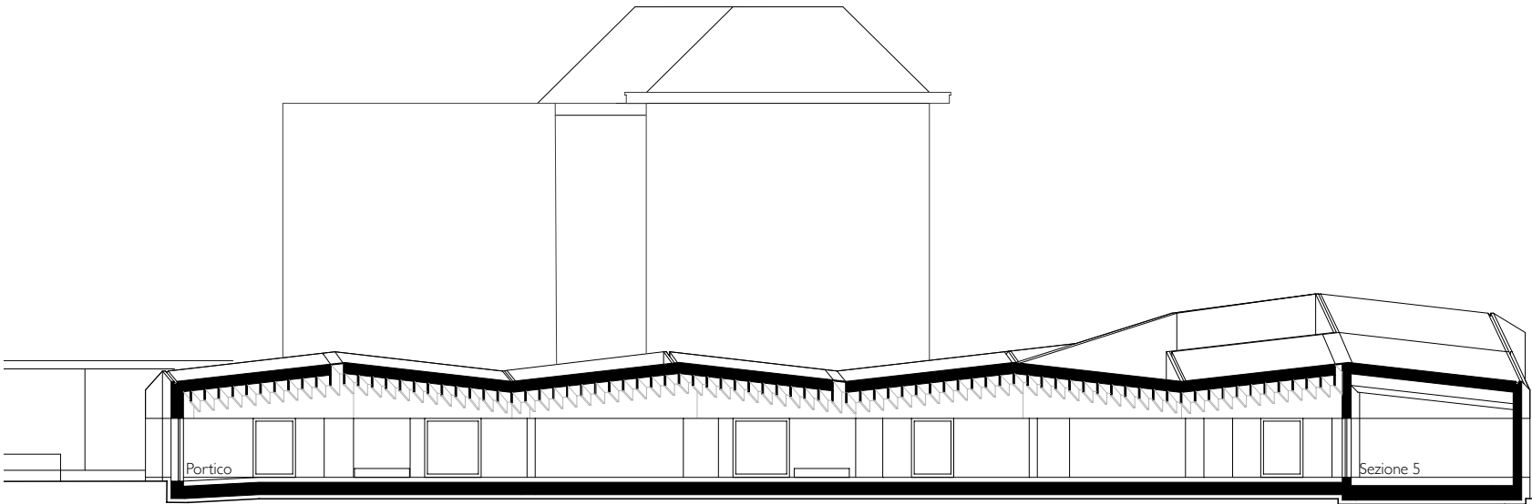
Sezione CC
