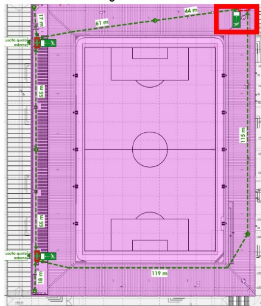
Schema delle vie di fuga del tetto con inserimento del nuovo corpo scala
