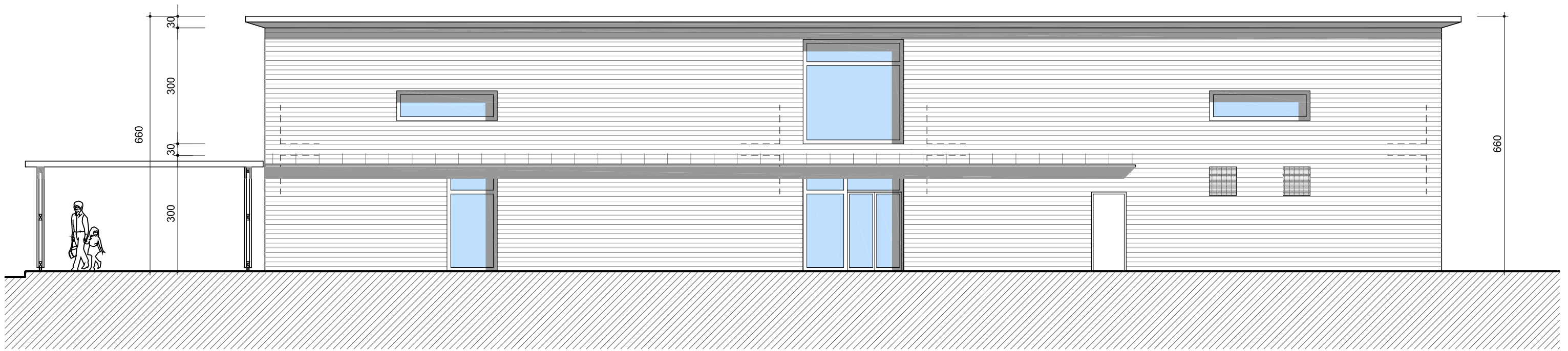
FACCIATA NORD-OVEST
